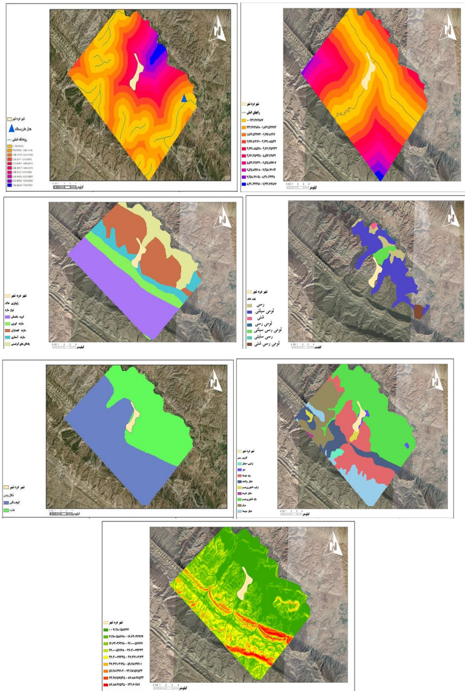
شکل (۲). لایه‌های اطلاعاتی دفن پسماند شهر دره‌شهر (منبع: تصاویر ماهواره‌ای و یافته‌های پژوهش)
